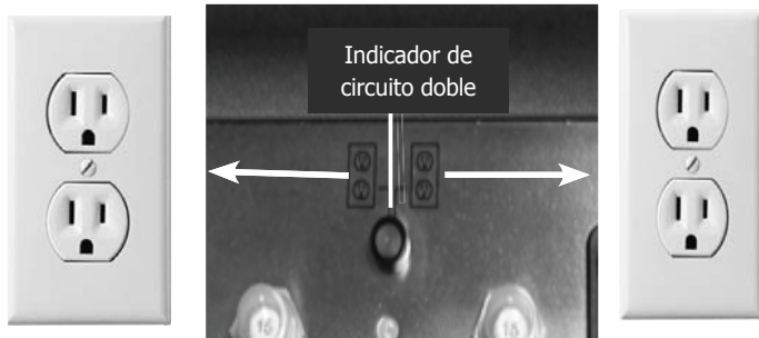
Circuito 2
